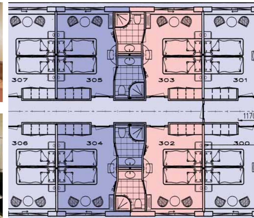
Kabinengrundriss Oberdeck (Mitteldeck)
